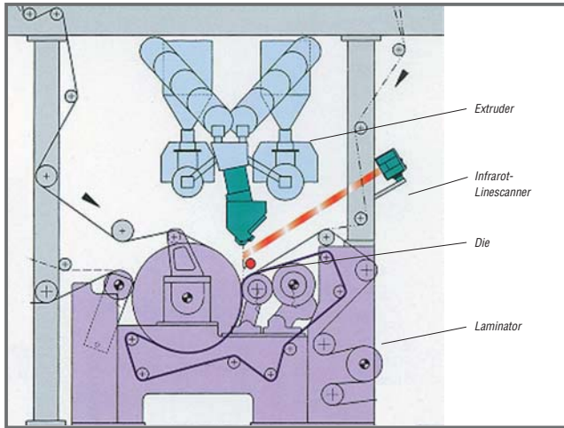
Beschichtungsprozess an einer Extrusionsanlage (Bild: mit freundlicher Genehmigung der EC-Erdölchemie)
