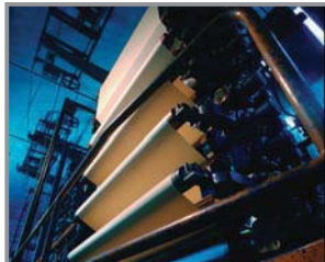
Bei der Herstellung von Papier überwachen Infrarotthermometer der Serie Thermalert den Trocknungsprozeß. Das Ergebnis: höherer Ertrag, geringere Stillstandszeiten.
